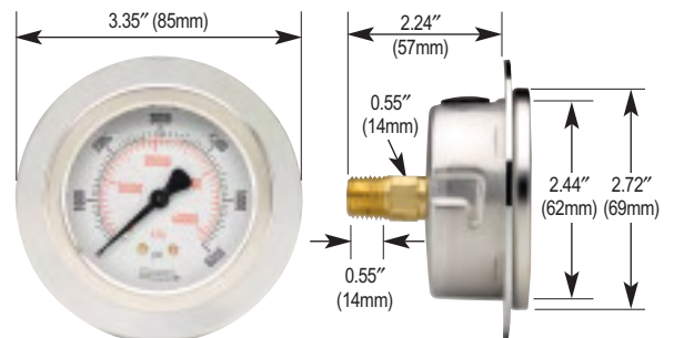
25-911 Flange Ring
