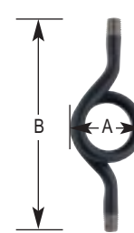
360° Syphon
