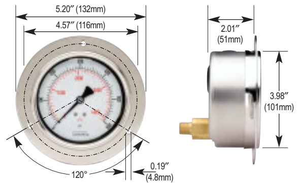
25-911 Flange Ring
